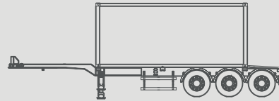
Ağır 20 ft Konteyner / Heavy 20 ft Container
