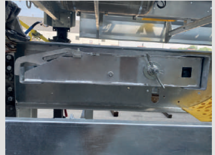
Konteyner Kilit Tutucu / Winglock Holder
